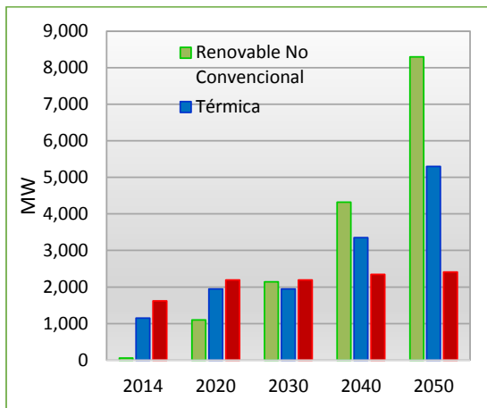
Gráfica N° 99. Capacidad Instalada por Tipo de Planta
