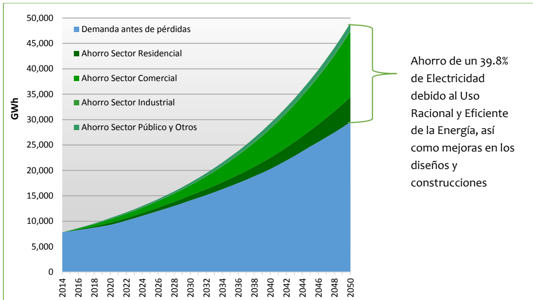
Gráfica N° 108. Efecto de la mejora en la eficiencia de Equipos y diseños en la demanda eléctrica
